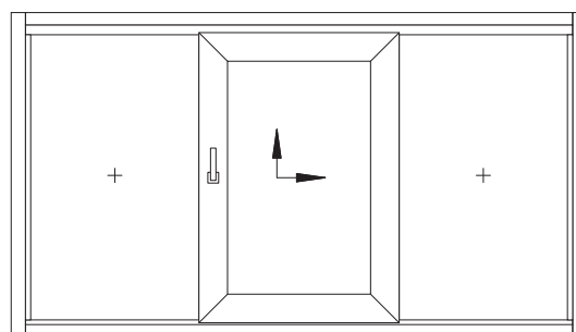
Jedno pohyblivé křídlo prostřední, s otevíráním doprava
