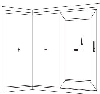
90° celoskleněný roh, jedno pohyblivé křídlo, s otevíráním doleva
